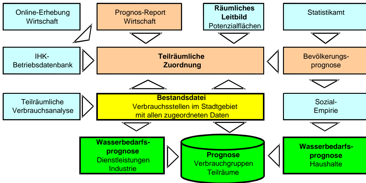
Abbildung 2: Datenverknüpfung für Analyse und Prognose
