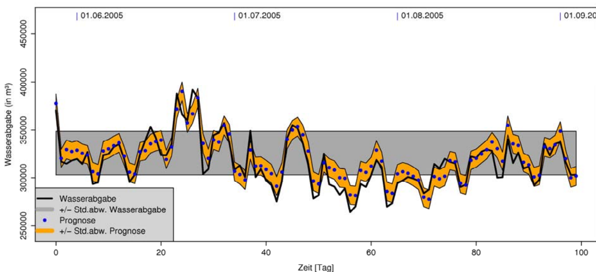
Abbildung 4: Prognose der täglichen Wasserabgabe in einem Zeitfenster von etwa drei Monaten (Beispiel Hamburg)
